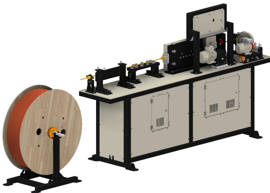
نمای کلی ماشین صاف کن و برش دیسکی مدل CTC-202-02
