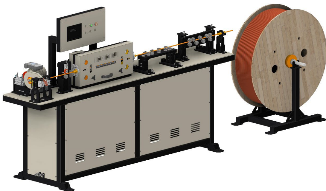
نمای کلی ماشین صاف کن و برش دیسکی مدل CTC-202-02
