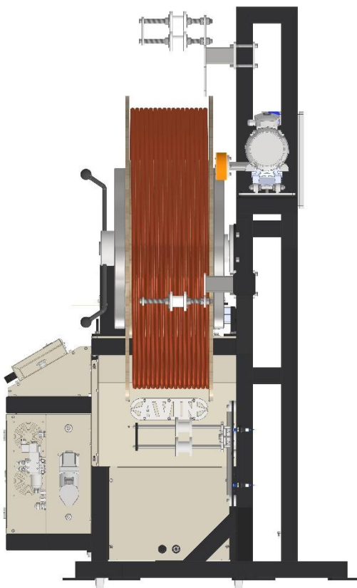
نمای کلی ماشین صاف کن و برش دیسکی مدل CTC-202-04
