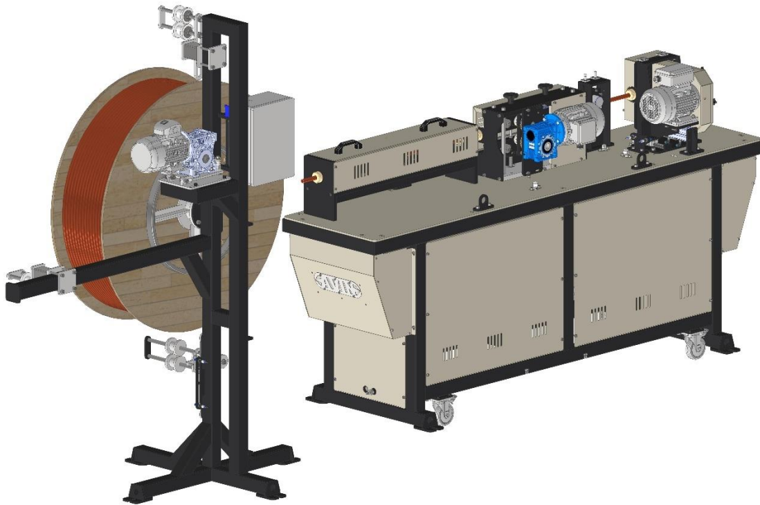
نمای کلی ماشین صاف کن و برش دیسکی مدل CTC-202-04
