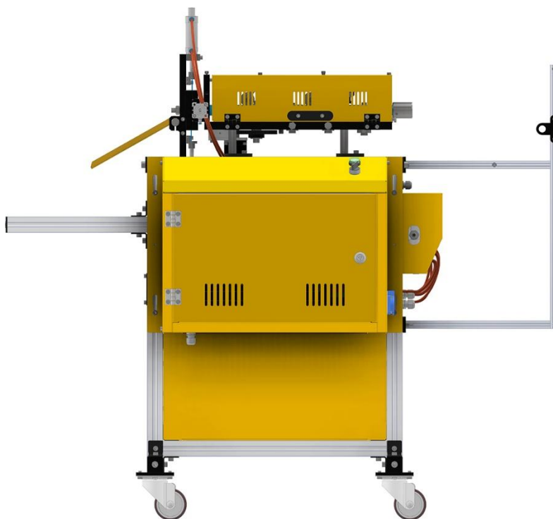
نمای جانبی ماشین برش اتوماتیک شلنگ خرطومی قلیان مدل FTC-103-02
