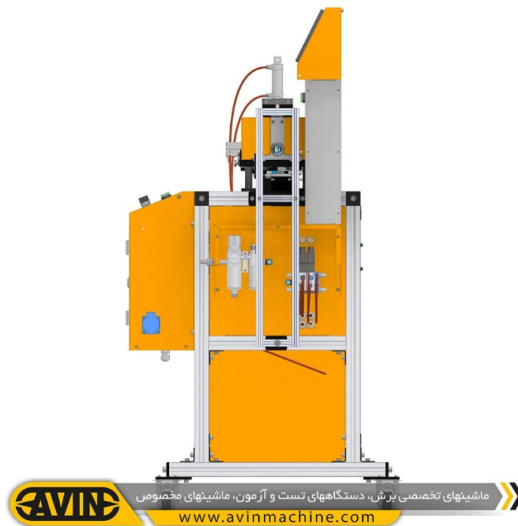
نمای پشت ماشین برش اتوماتیک شلنگ قلیان مدل FTC-103-03
