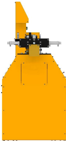
نمای جلو ماشین برش اتوماتیک شلنگ خرطومی قلیان مدل FTC-103-04
