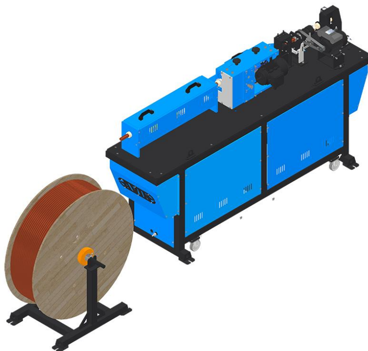
نمای ایزومتریک ماشین برش اتوماتیک لوله مسی مدل CTC-104-02
