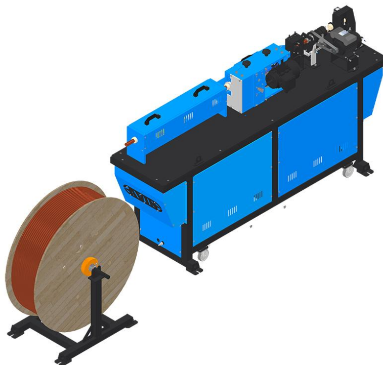
نمای ایزومتریک ماشین برش اتوماتیک لوله مسی مدل CTC-104-03
