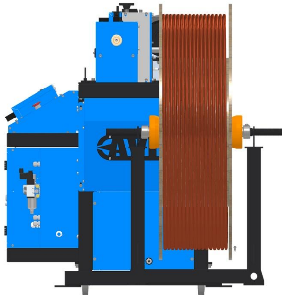
نمای پشت ماشین برش اتوماتیک لوله مسی مدل CTC-104-03
