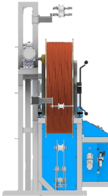
نمای پشت دستگاه برش حرفه‌ای لوله‌های مسی مدل CTC-105-02
