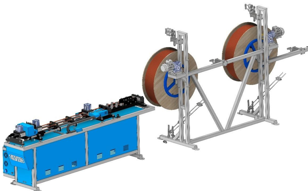
نمای ایزومتریک دستگاه برش حرفه‌ای لوله‌های مسی مدل CTC-105-02
