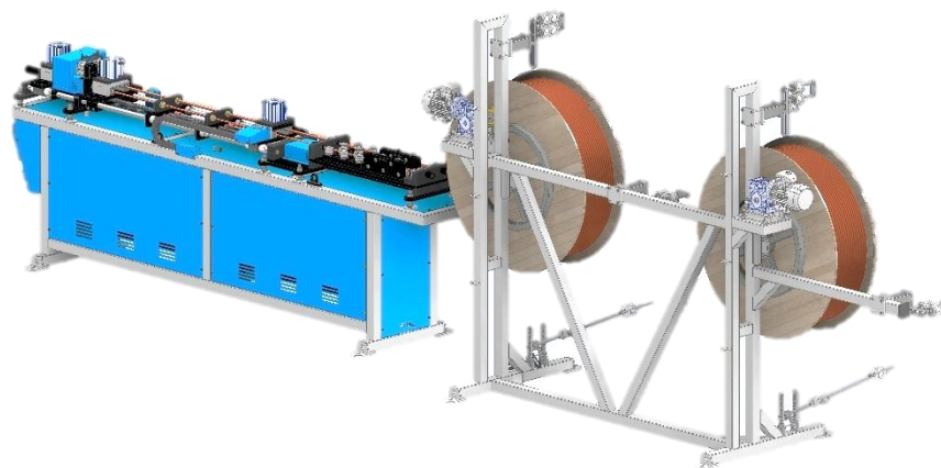
نمای ایزومتریک دستگاه برش حرفه‌ای لوله‌های مسی مدل CTC-103-02
