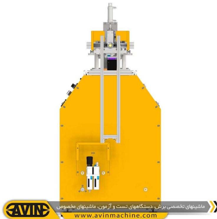
نمای جلو ماشین برش اتوماتیک شلنگ خرطومی قلیان مدل FTC-103-01
